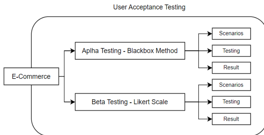
Gambar 2. Pengujian UAT
