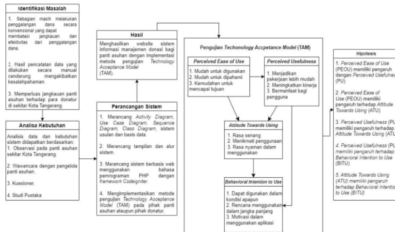
Gambar 1. Kerangka Penelitian
