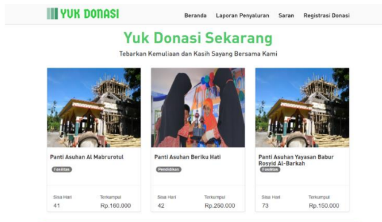
Gambar 3. Halaman Donatur
