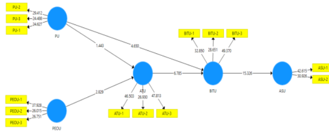
Gambar 8. Hasil Bootstrapping dengan aplikasi SmartPLS
