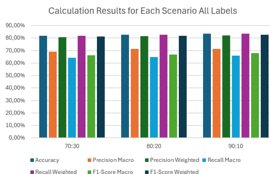
Gambar 3. Penerapan Naïve bayes
