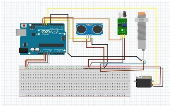
Gambar 8. Rangkaian Keseluruhan
