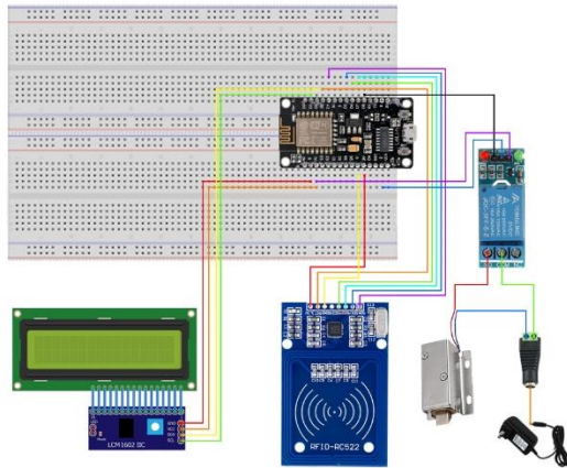
Gambar 6. Rangkaian Mikrokontroler Utama
