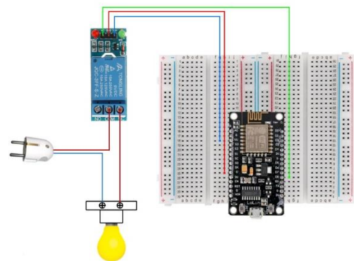
Gambar 7. Rangkaian Mikrokontroler Lampu
