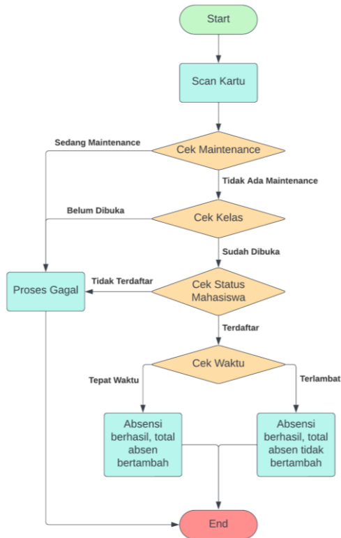
Gambar 1. Flowchart Mahasiswa
