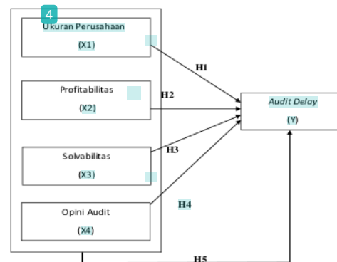
Gambar 1. Kerangka Pemikiran
