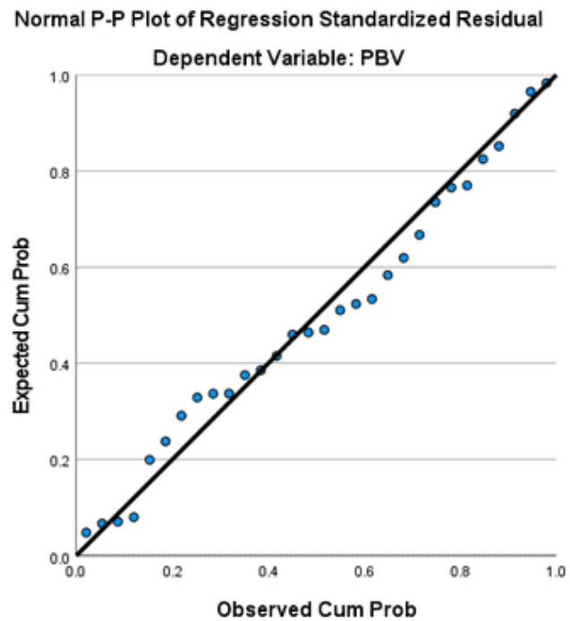
Gambar IV.2 Hasil Uji Normalitas P-P Plot
