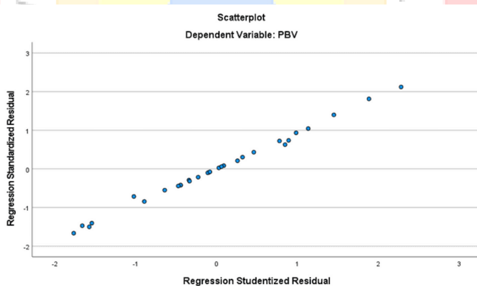
Gambar IV.3 Hasil Uji Heteroskedastisitas
