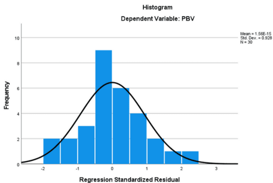
Gambar IV.1 Hasil Uji Normalitas Grafik Histogram
