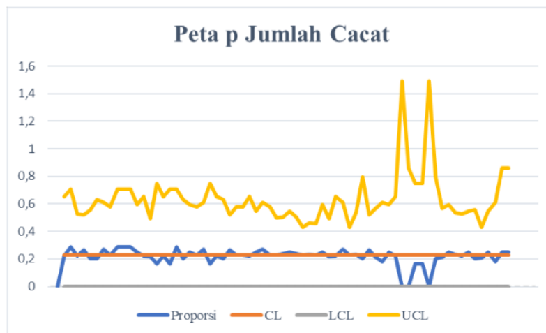
Gambar 2. Peta p Jumlah Cacat
