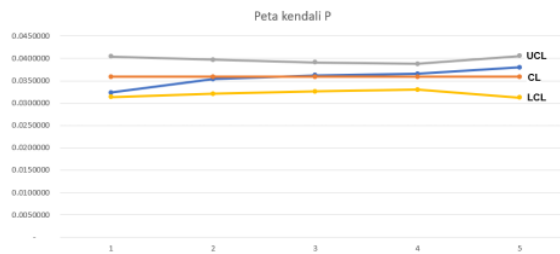
Gambar 2. Peta p kain spun polly periode Agustus 2023 setelah revisi
