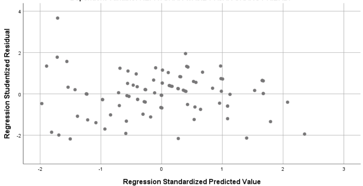
Dependent Variable: KEPATUHAN WAJIB PAJAK ORANG PRIBADI
